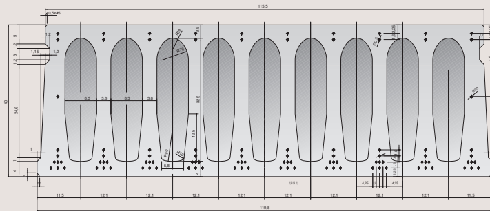
f forjado placa alveolar de 120 x 40 cm.
