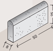
c bordillo jardín bicapa
