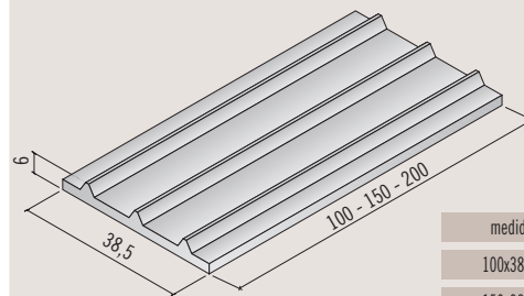
e placa cubierta ancho 0,385 m.
