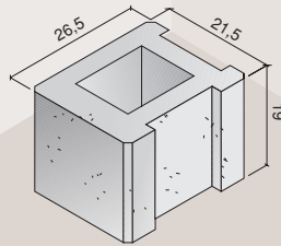
d esquina b-12
