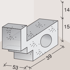
a cornisa Lillo
