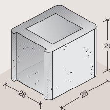
j 1 encaje b-20
