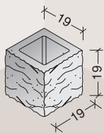
c medio term. sp. 20
