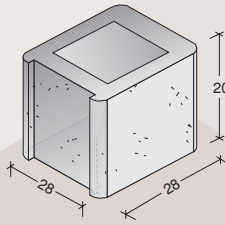
f 1 encaje b-15
