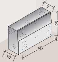
b bordillo A2 bicapa
