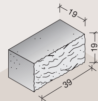
b sólido split
