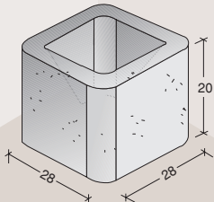
e standard b-15
