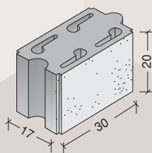
i acústico 30 x 20 x 17
