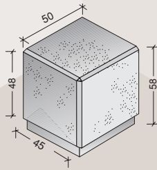
b cubo hormigón 0,50 m.
