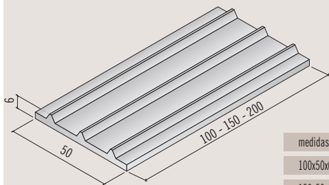
d placa cubierta ancho 0,50 m.
