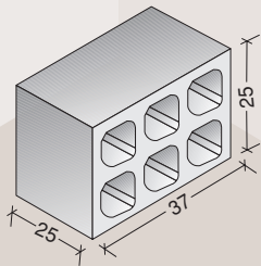
e botellero arlita
