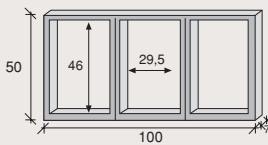
h 1 hueco 0,50 x 0,25 m / 0,50 x 0,33 m / 0,50 x 1 m
