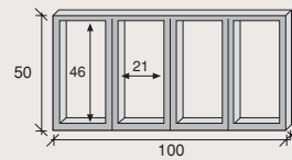
g 4 huecos 1 x 0,5 m
