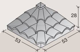
t sombrero granadino
