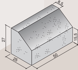
e bordillo isleta alto
