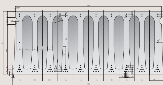
g forjado placa alveolar de 120 x 50 cm.
