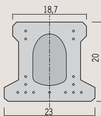
h viga tubular canto 20 cm.
