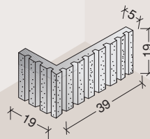
k pieza en "L" rudolph
