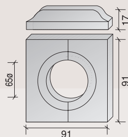
f alc. 91x91 ø65
