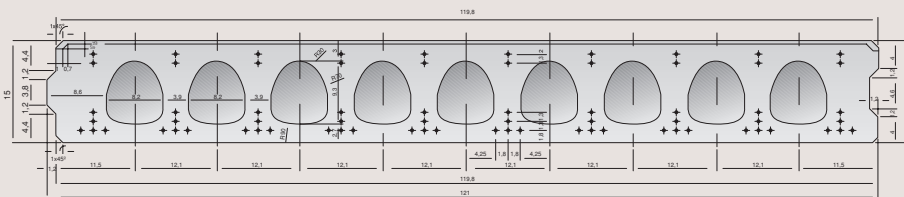
b Placa alveolar de fachada Rocés de acabado visto
