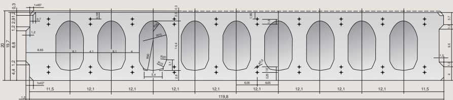
c Placa alveolar de fachada Rocés de acabado visto
