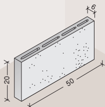
a tabiquero de arlita
