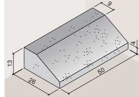
d bordillo isleta bajo
