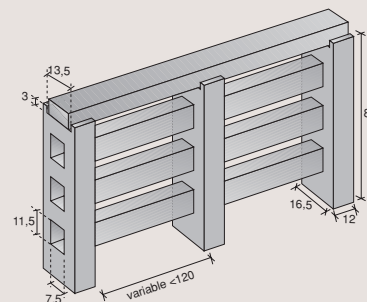
g poste modelo Vega
