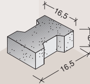
b "H" modelo 2 bicapa
