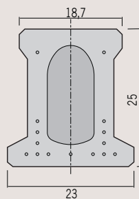
i viga tubular canto 25 cm.
