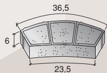
e Coda modelo 6 bicapa
