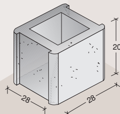
k 2 encajes b-20
