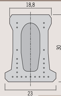
j viga tubular canto 30 cm.
