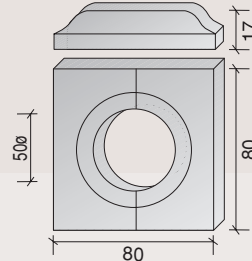
g alc. 80x80 ø50
