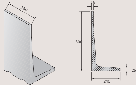
b separador graneles "L" 5 m.
