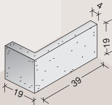
i pieza en "L" std.
