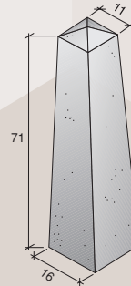
g hitos de hormigón
