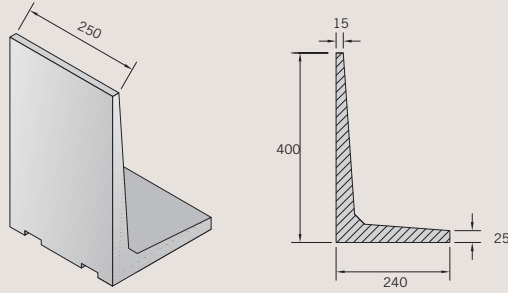
a separador graneles "L" 4 m.
