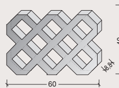
g celosía césped
