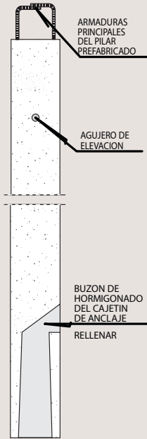
SECCION POR BUZÓN
