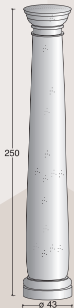
a c. de orden toscano
